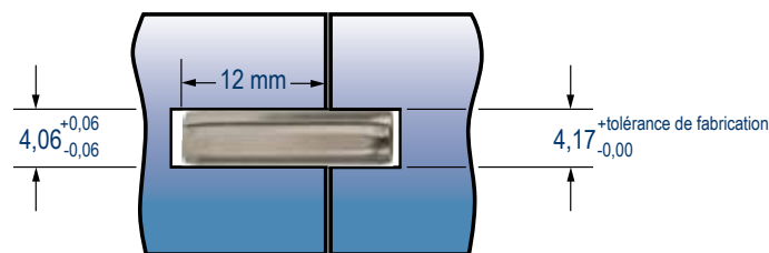
Taille du trou recommandée pour ajustement avec jeu avec CLDP 4 x 20 LBK
