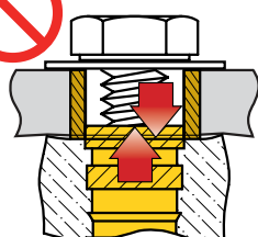
Arrachement
