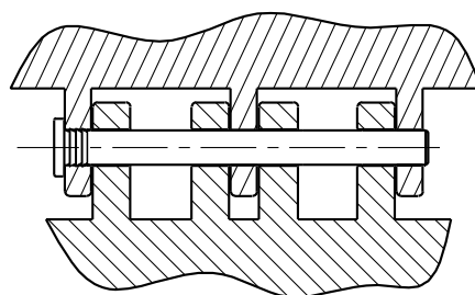
Exemple d'application : Goupille Loquet dans une poignée de portière de voiture
