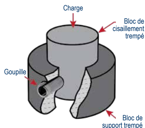
Test de cisaillement effectué dans un montage selon ISO 8749
